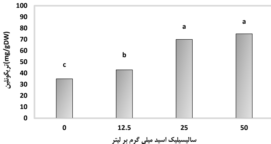
شکل 4. اثر سالیسیلیک‌اسید بر میزان تریگونلین. مقادیر نشان داده شده میانگین سه تکرار می‌باشد. (میانگین‌های دارای حرف مشترک از نظر آماری در سطح 5 درصد تفاوت معنی‌داری ندارند.)
