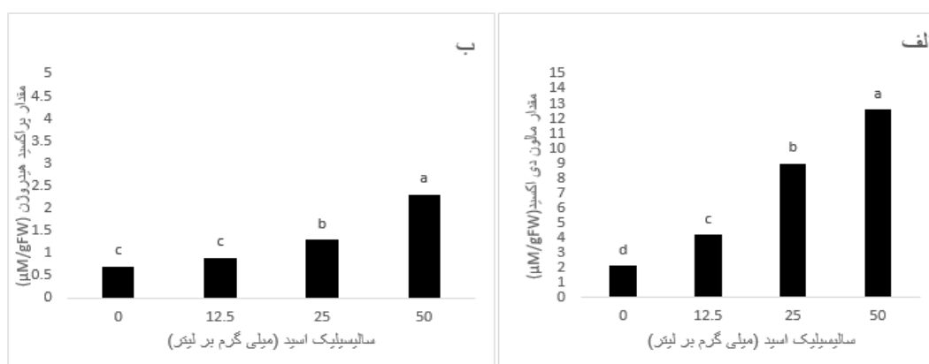
شکل 2. اثر سالیسیلیک‌اسید بر (الف) مقدار مالون‌دی‌اکسید، (ب) مقدار پراکسید هیدروژن در کشت سلولی شنبليله. میانگین سه تکرار است. (میانگین‌های دارای حرف مشترک از نظر آماری در سطح 5 درصد تفاوت معنی‌داری ندارند).
