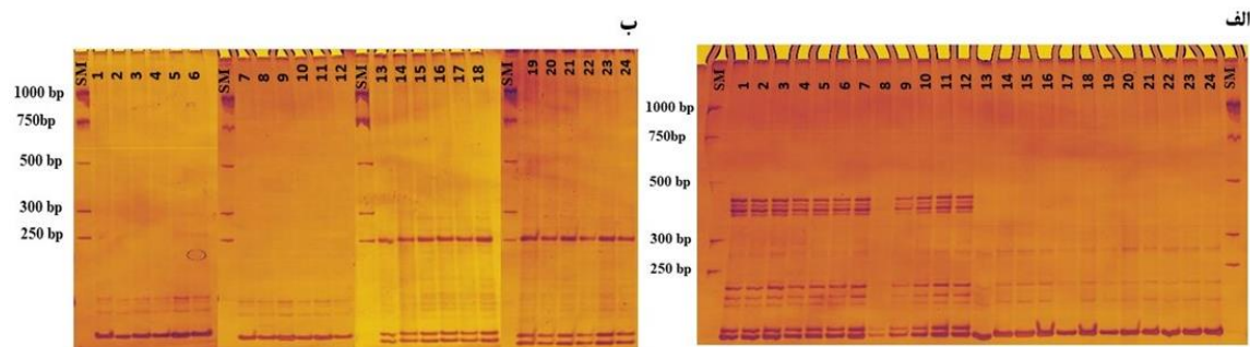
شکل ۱. الگوهای باندی نشانگر SSR در دو رقم سیب‌زمینی (آریندا و سانته) تکثیر شده با آغازگر STI0014 (الف) و STM1104 (ب) روی ژل پلی‌آکریل‌آمید ۱۰ درصد. SM: نردبان مولکولی، ترتیب نمونه‌ها عبارتند از: شماره ۱-۳: ریزنمونه‌های سانته (نگهداری غیر فراسرد)، شماره ۴-۶: ریزنمونه‌های سانته (نگهداری فراسرد)، شماره ۷-۹: گیاهان نسل اول سانته (نگهداری غیر فراسرد)، شماره ۱۰-۱۲: گیاهان نسل اول سانته (نگهداری فراسرد)، شماره ۱۳-۱۵: آریندا (نگهداری غیر فراسرد)، شماره ۱۶-۱۸: آریندا (نگهداری فراسرد)، شماره ۱۹-۲۱: گیاهان نسل اول آریندا (نگهداری غیر فراسرد) و شماره ۲۲-۲۴: گیاهان نسل اول آریندا (نگهداری فراسرد). همان‌طور که در شکل مشخص است باندهای حاصله کاملاً مشابه هستند.
