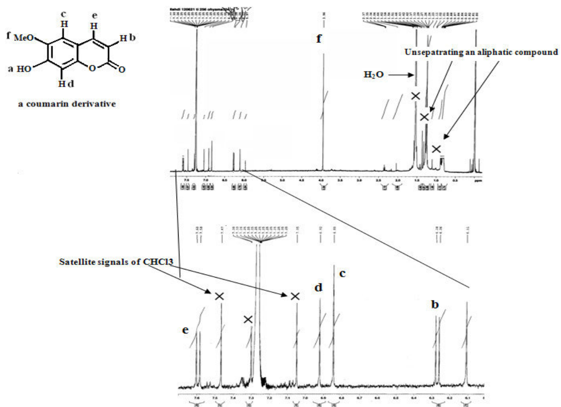
شکل ۴- ^1\text{H-NMR} ترکیب فلورسانس استخراج شده از سلول‌های کشت سوسپانسیون زیره سیاه
