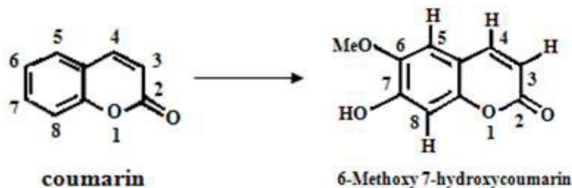
شکل ۵- ساختار کومارین و ترکیب فلورسانس استخراج شده از سلول‌های کشت سوسپانسیون زیره سیاه
