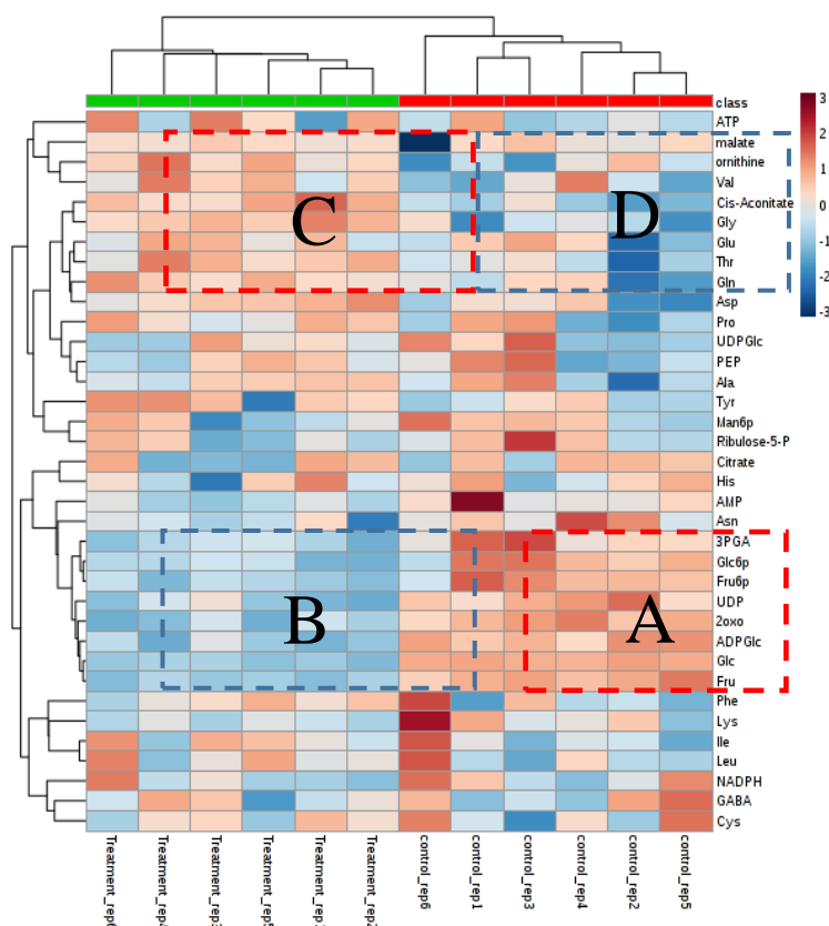
شکل ۳. نقشه حرارتی پروفایل متابولیت‌ها و آمینواسیدها در نمونه‌های کنترل و تیمار شده با آلومینیوم. در بالای شکل رنگ قرمز نشان‌دهنده گروه کنترل و رنگ سبز نشان‌دهنده گروه تیمار شده با آلومینیوم است. تعداد شش تکرار در هر گروه مورد استفاده قرار گرفت. محدوده شدت رنگ از +۳ تا -۳ فراوانی نسبی هر ماده را به ترتیب از فراوانی زیاد (قهوه‌ای) به فراوانی کم (آبی) نشان می‌دهد. حروف A تا D بیانگر گروه‌های تفکیک‌شده‌ای از متابولیت‌ها در نمونه‌های کنترل و تیمار است.
